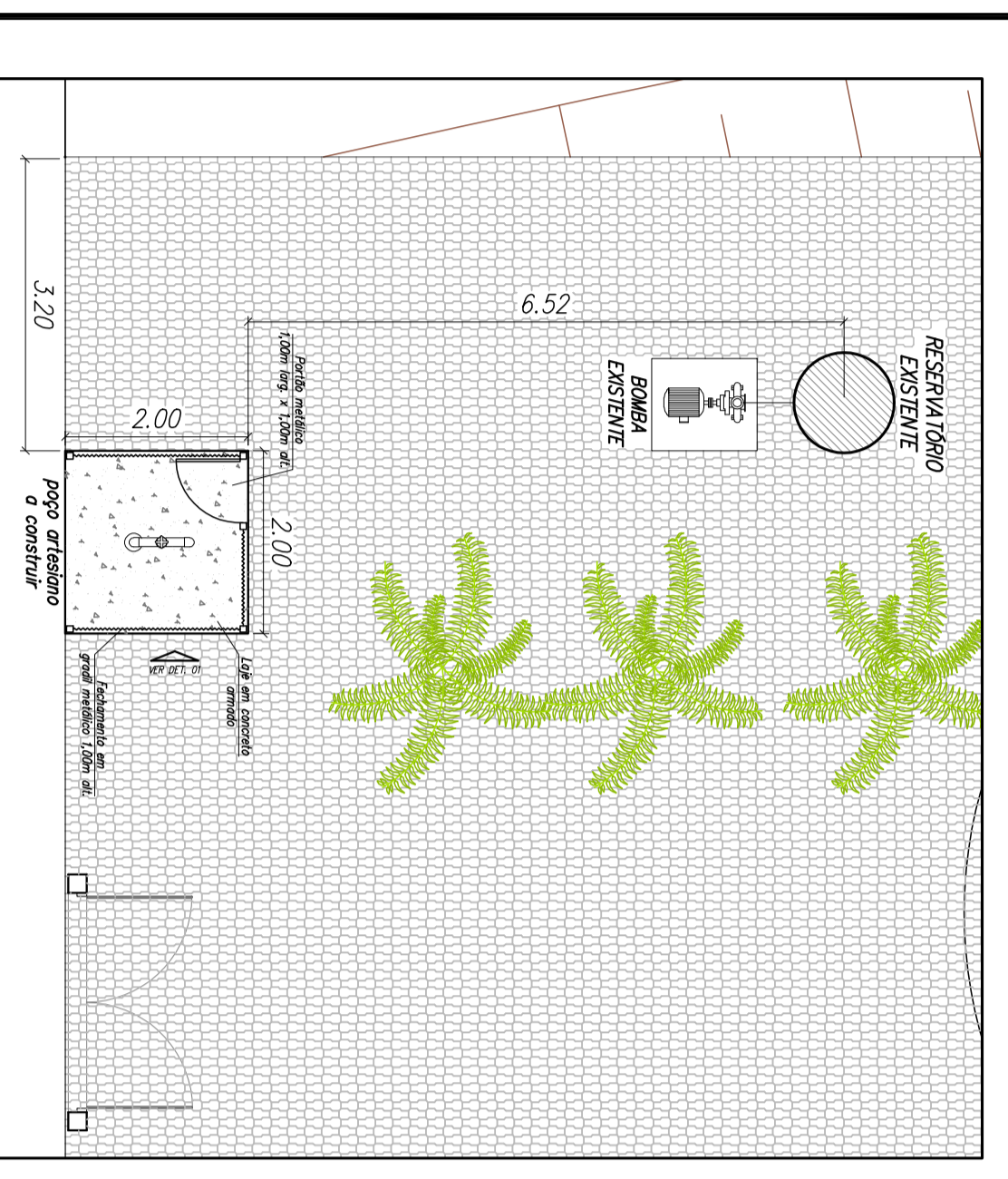
IMPLANTAÇÃO POÇO ARTESIANO ESCALA 1:75
